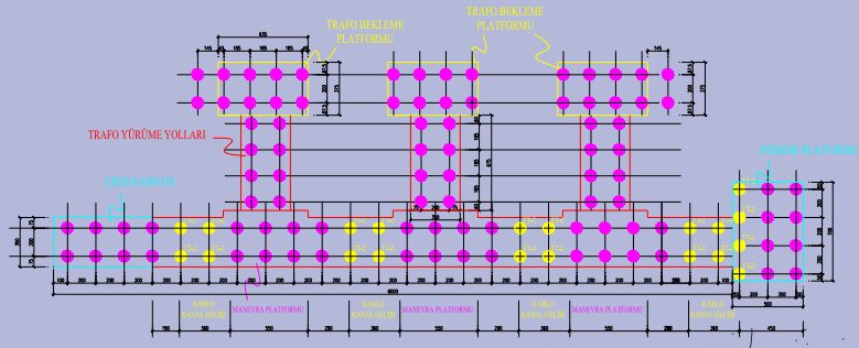
TRAFO BEKLEME PLATFORMU, MANEVRA PLATFORMU, İNDIRME PLATFORMU VE YÜRÜME YOLLARI JET-GROUT APLİKASYON PLANI
